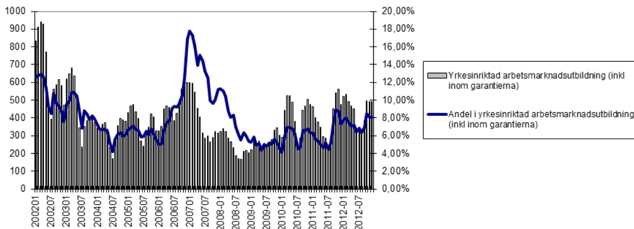
Antal och andel* i yrkesinriktad arbetsmarknadsutbildning, inkl. garantierna, Norrbottens län, 2002-2012
